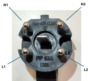
Perilex Din 49446 2P + 2N 16A Kookgroep
