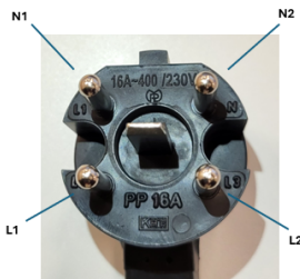
Perilex Din 49446 2P + 2N 16A Kookgroep
